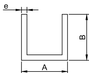
Perfil U
